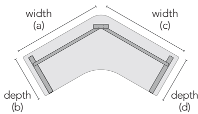
3 leg 120°
